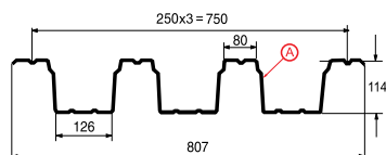
Профилированный лист H-114x750-A
