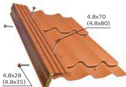
Продольное перекрывание 1 волна
