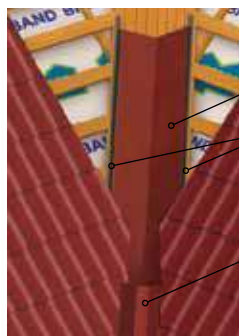
Планка ендовы нижняя Уплотнитель Планка ендовы верхняя
