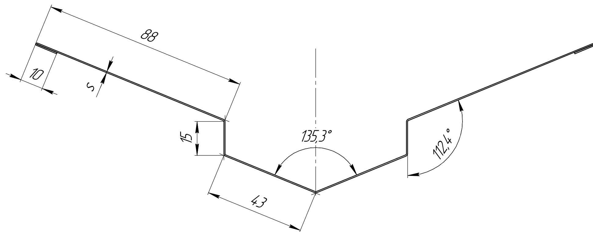
Планка ендовы верхней 88x43x43x88
